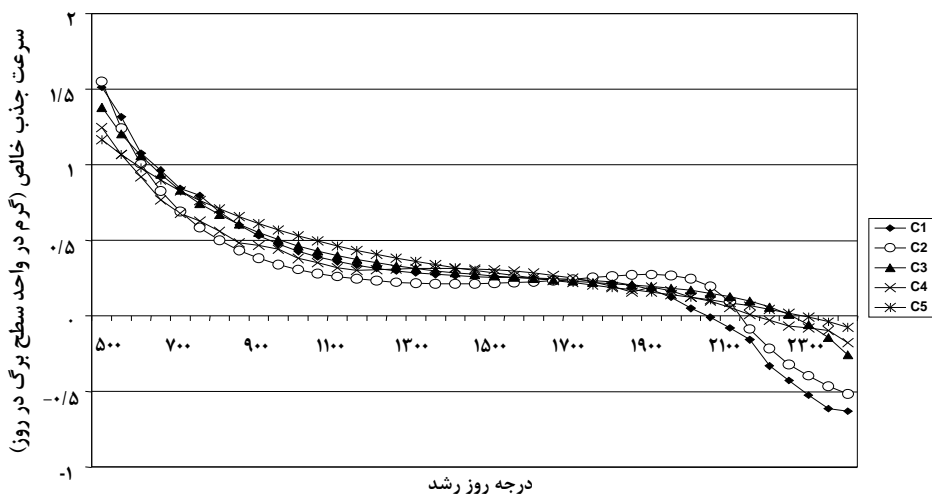
شکل ۲- روند تغییرات سرعت جذب خالص گیاه ماش تحت تأثیر مقادیر مختلف کمپوست.
