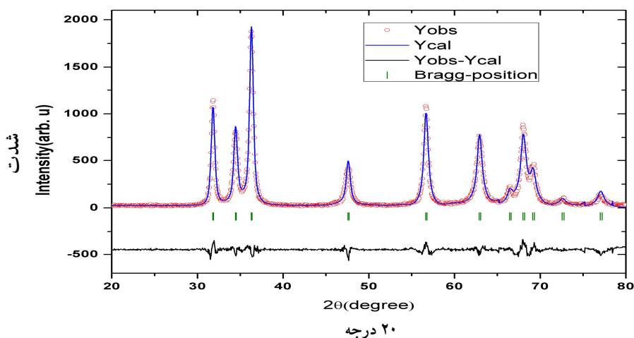
شکل ۱- الگوی XRD و خلوص Rietveld نانوذرات اکسید روی سنتز شده.
