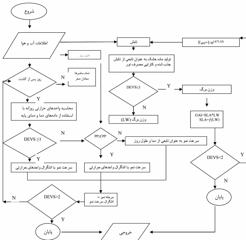
شکل ۲- الگوریتم مدل CUMMOD. اختصارات عبارتند از: F_{abs} (کسر جذب نور)، DEVS (مرحله نمو)، K (ضریب خاموشی نور)، SGA (سطح سبز ویژه)، GLA (سطح برگ سبز). Y و N هم تایید و عدم تایید شروط الگوریتم را نشان می‌دهند.
